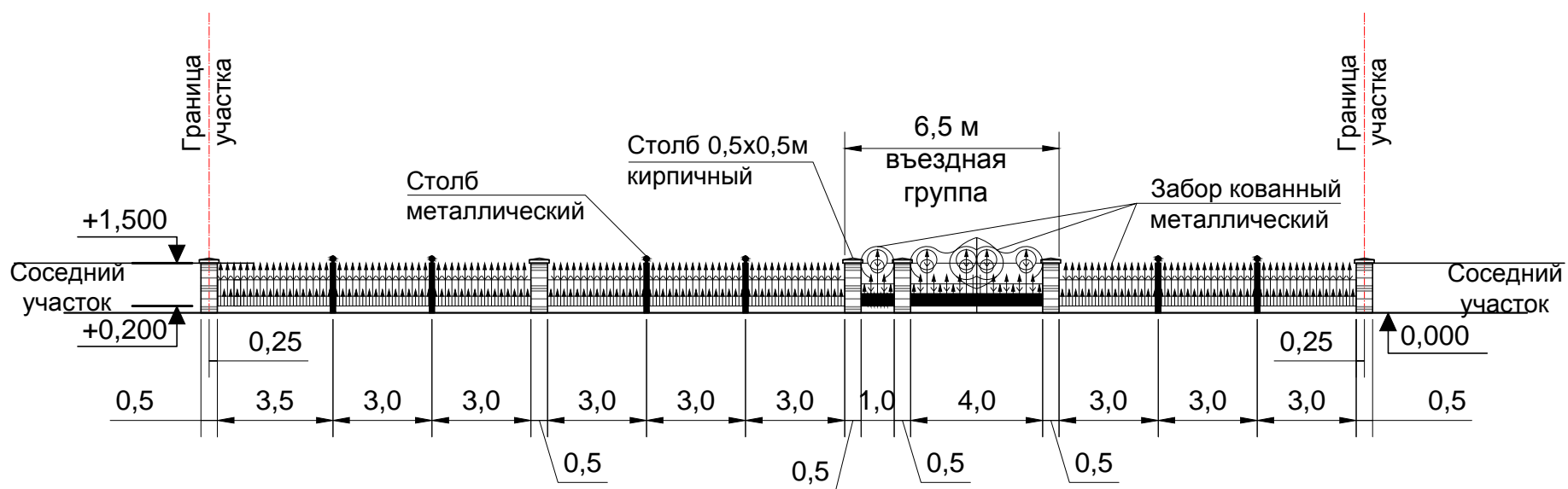
Вид А
